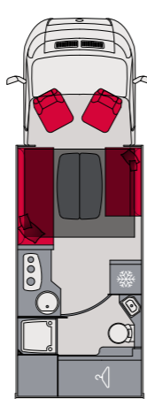
P696D D pour dressing (sans lit permanent)
