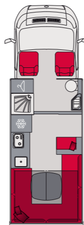
P696U U pour salon en U (sans lit permanent)
